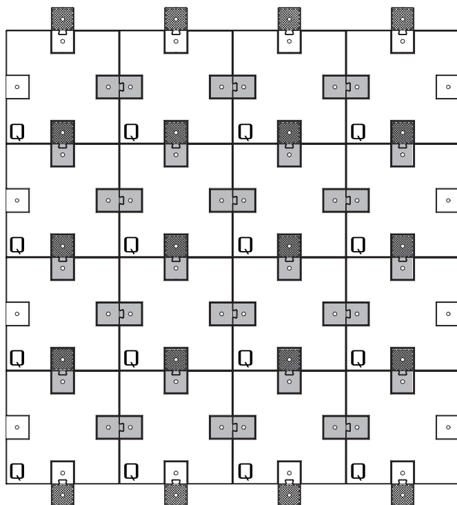
Sistema di Montaggio SUPERFICIALE
